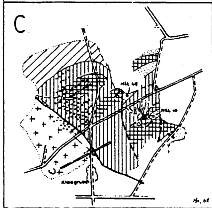
Abb. 1. Kartierungen am Eichberg bei Weifig. — A: K. PIETZSCH 1907 (Ausstrich + Lesesteine), B: G. HERBST u. a. 1958, Originalmaßstab 1 : 10 000, Störungen zwischen Granit und Silur nach PIETZSCH ergänzt, Kartierung der Störung durch ANDERS 1962, C: nach BRAUSE 1969 (Geländeaufnahmen: G. HIRSCHMANN & H. BRAUSE 1961/1962). — 1 = Granit, 2 = Silur, allgemein, 3 = Silur, vorwiegend Kieselschiefer, 4 = Eichbergsandstein (oberes Ordovizium), 5 = sonstiges Paläozoikum, 6 = Störung, sicher / vermutet, 7 = morphologischer Gehängeknick, 8 = Graptolithenfundpunkt, 9 = starke Quarzdurchtrümmung, 10 = Schürfe, 11 = Bohrpunkt.
