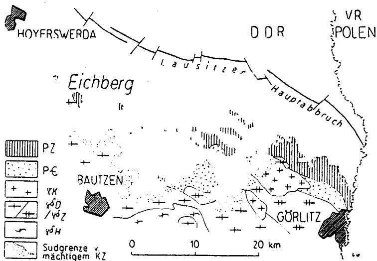
Karte 1. Lageübersicht. — PZ = gefaltetes Paläozoikum, PE = Präkambrium, Lausitzer Grauwackeneinheit, \gamma K = Königshainer Stockgranit, \gamma\delta f = Demitzer Granodiorit, \gamma\delta z = Seidenberger Granodiorit, \gamma\delta H = Hybridgranodiorit, KZ = Känozoikum.
