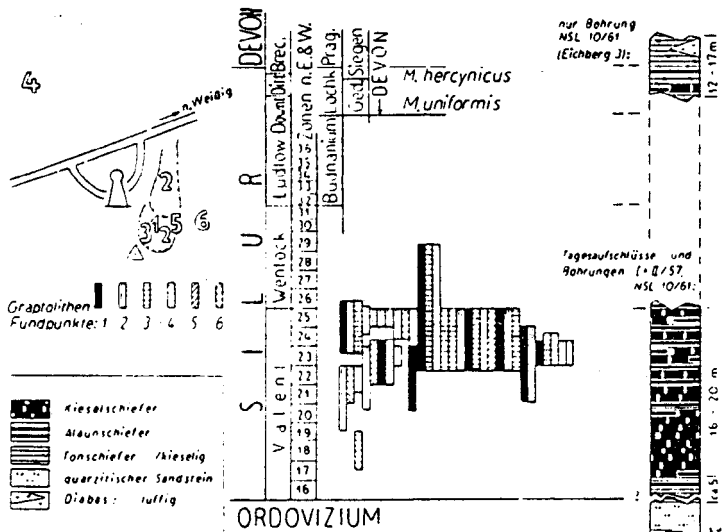
Abb. 3. Stratigraphische Verbreitung der vom Eichberg bekannten Graptolithenarten und schematisches Silur-Normalprofil vom Eichberg. Fundpunkte: 1 = nach PIETZSCH 1962, Tab. S. 185, 2 = nach H. GRUHL 1955, S. 190, 3 = neue Aufsammlungen im oberen Steinbruch, 4 = Fund auf den Feldern nördlich des Denkmals, 5 = Bohrungen Eichberg I + II 57, 6 = Bohrung NSL 10 61 (Eichberg 3); Bestimmungen bei 3–6 von G. FREYER.
